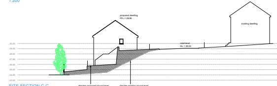
SITE SECTION C-C 1:200
